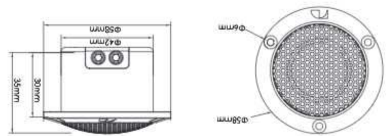
Dimensions (Unit:mm)
